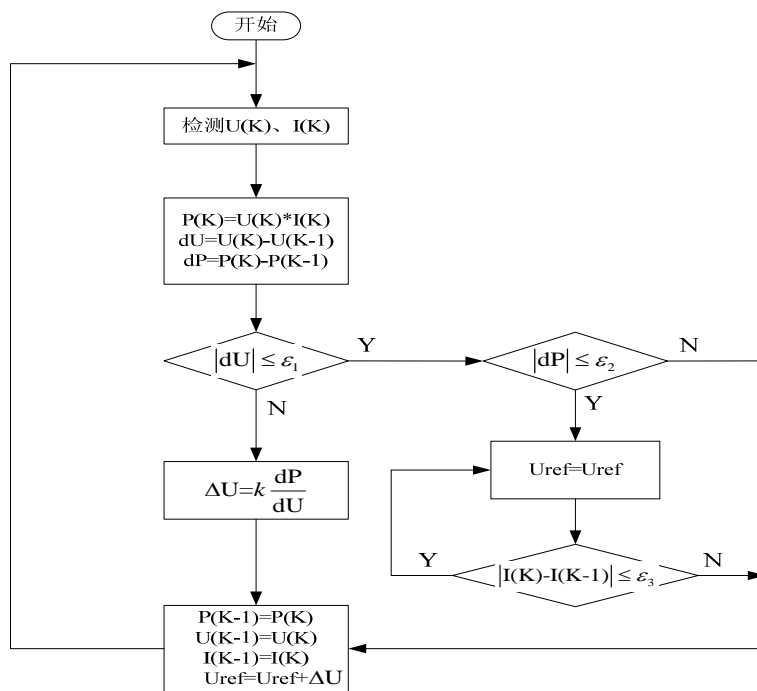
图 5: MPPT 流程图
