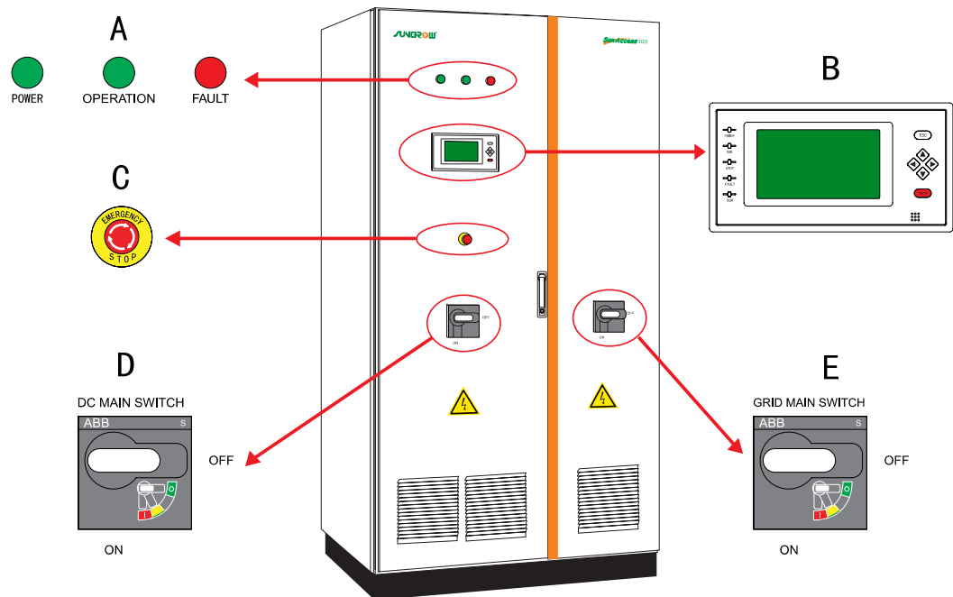
图3-6 SG100K 外观图
